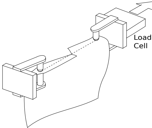
Figura 3.3: Diagrama del montaje experimental utilizado en el experimento de O'keefe, se observa que los soportes tienen extremos esféricos para que las solapas puedan girar en los puntos de tiro
