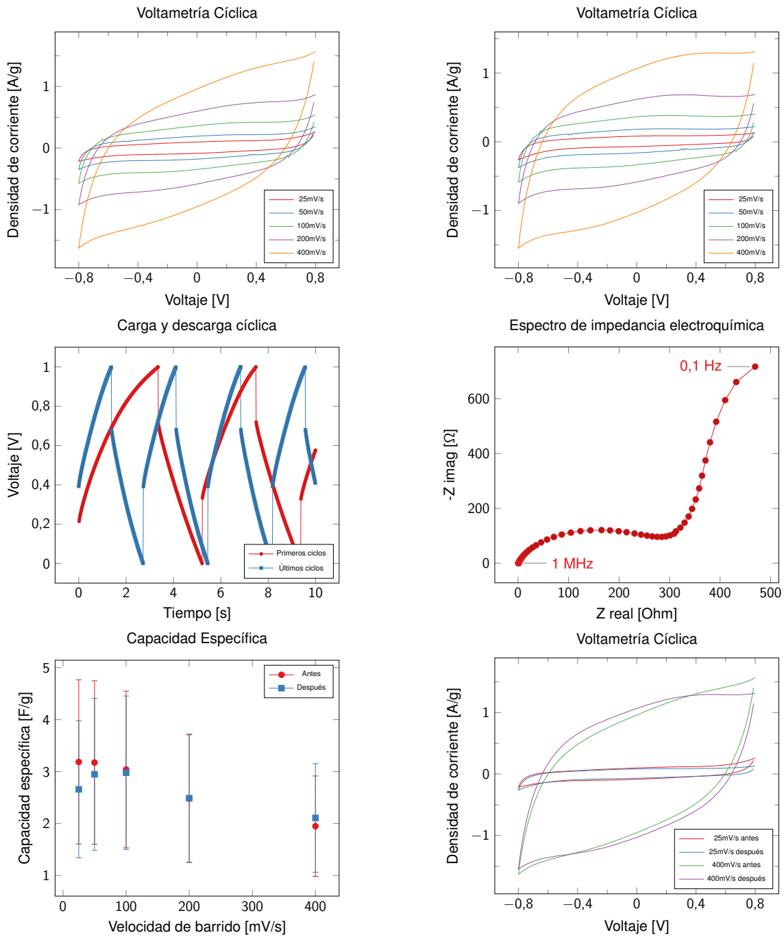
Figura A.4: Polvo en disco de acero. Masa = 0.4 mg.
