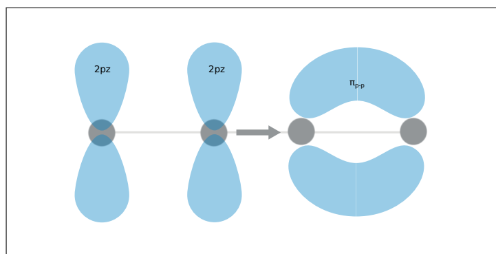
Figura A.2: Vista lateral de grafeno. Formación de un orbital \pi_{p-p} entre dos átomos de carbono. Junto con el orbital \sigma forman un enlace doble entre átomos de carbono.
