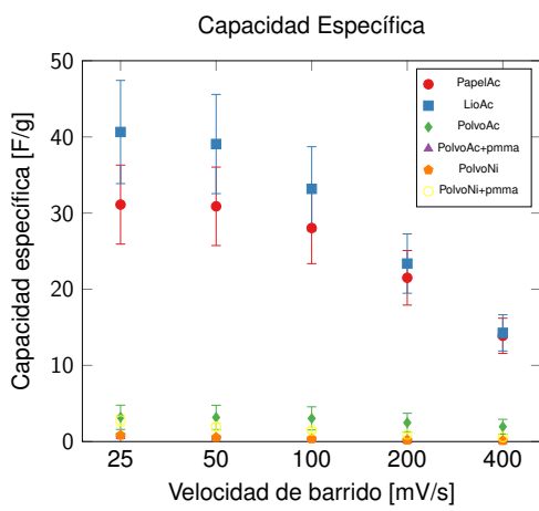
(a) Capacidad específica antes de 1000 ciclos de carga y descarga.
