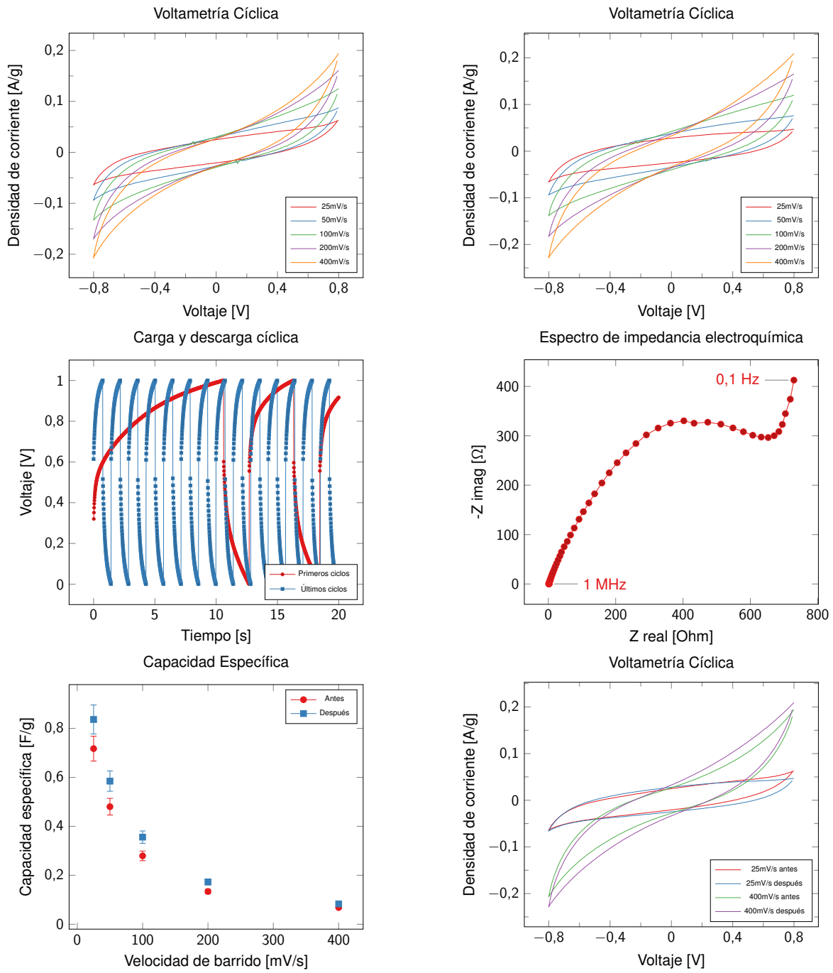
Figura A.5: Polvo + PMMA en disco de acero. Masa = 2.8 mg.
