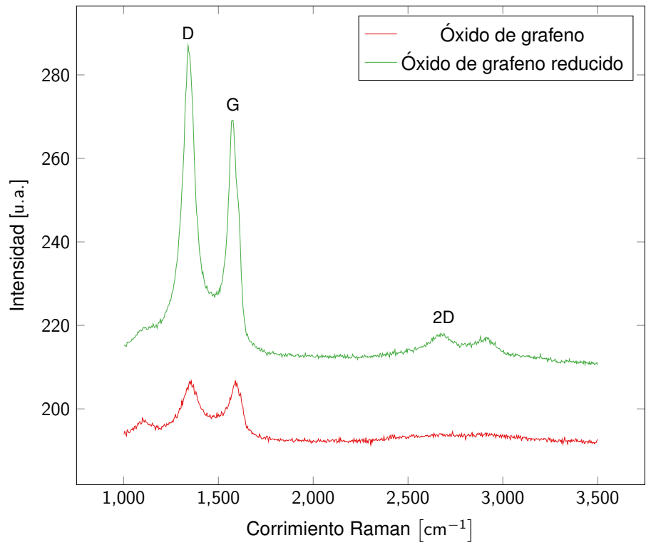
Figura 2.3: Espectro Raman de muestras de óxido de grafeno y óxido reducido de grafeno.
