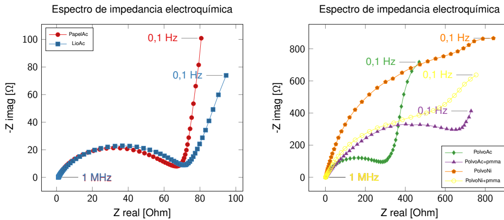
Figura 3.5: Resumen del espectro de impedancia electroquímica. Las muestras son separadas en dos gráficos para mejorar su visualización.
