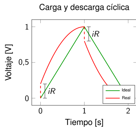
Figura 14: Ejemplo de carga y descarga.
