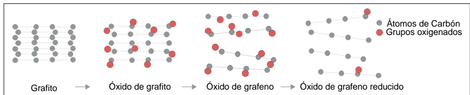
Figura 6: Síntesis de grafeno a través de la ruta del óxido de grafeno.
