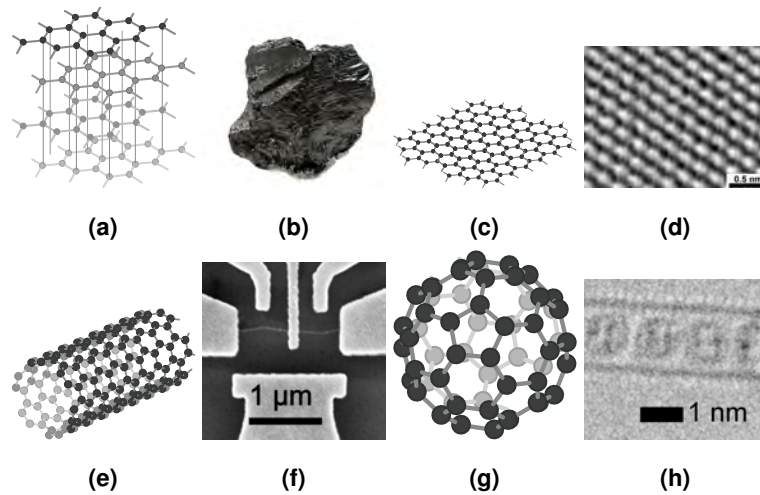
Figura 2: Estructuras e imágenes de varios alótipos del carbono como ejemplos de la dimensionalidad de los nanomateriales: (a) y (b) grafito natural, un material 3D. (c) y (d) grafeno, imagen de microscopía de efecto túnel (Frank Trixler, LMU/CeNS: Organic Semiconductor Group), un material 2D. (e) y (f) nanotubo de carbono, imagen SEM de un dispositivo para medir diferentes propiedades del nanotubo (Pavlos Apostolidis, London Centre for Nanotechnology, Department of Physics & Astronomy), un material 1D. (g) y (h) fullereno, imagen TEM de fullerenos C80 funcionalizados dentro de un nanotubo de carbono (Gimenez-lopez et al., 2011), un material 0D.
