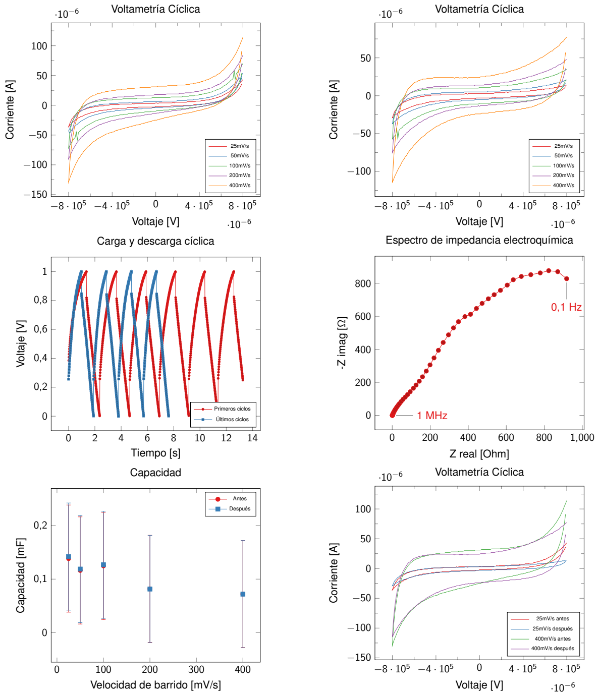
Figura A.3: Disco de acero sin material.
