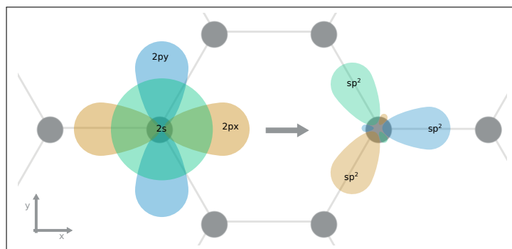
Figura A.1: Vista frontal. Hibridación sp 2 de los átomos de carbono del grafeno. Dos orbitales 2p, junto con el orbital 2s forman tres orbitales sp 2 que se disponen de forma planar con un ángulo de 120° entre ellos. Estos orbitales forman enlaces \sigma entre átomos de carbono.
