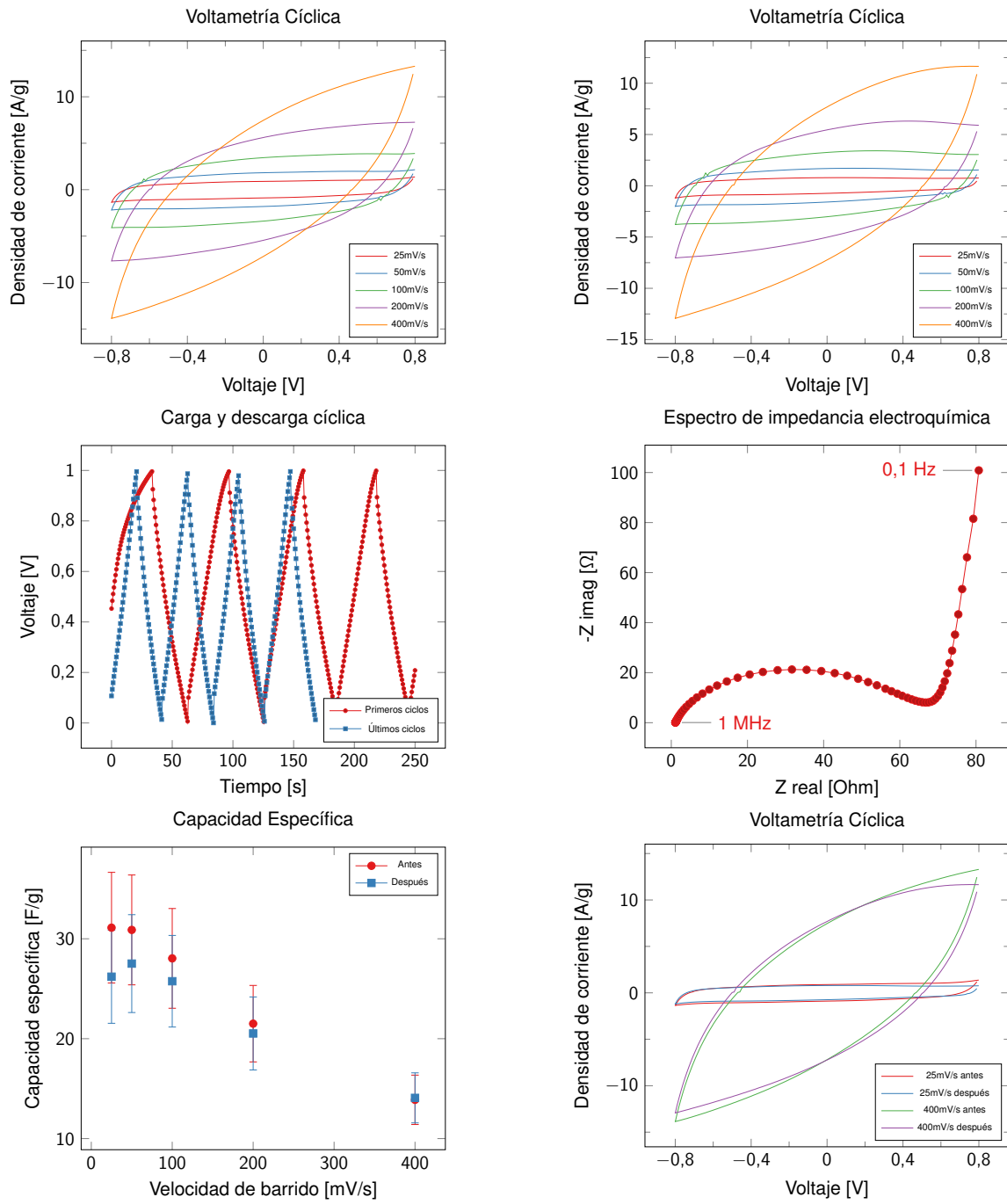
Figura A.6: Papel en disco de acero. Masa = 0.6 mg.
