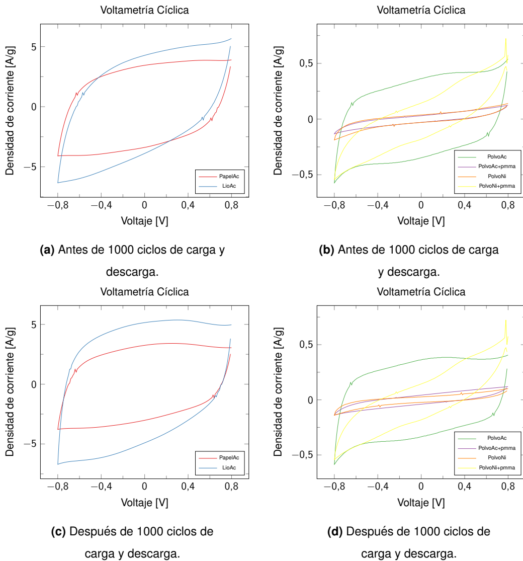
Figura 3.4: Resumen voltametría cíclica a 100 mV/s antes y después de 1000 ciclos de carga y descarga. Las muestras son separadas en dos gráficos para mejorar su visualización.
