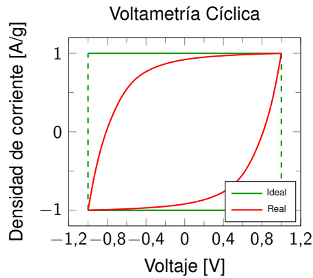
Figura 13: Ejemplos de voltametría cíclica.
