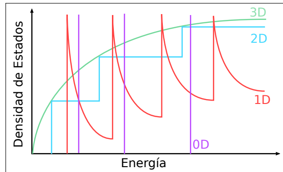
Figura 3: Densidad de estados en diferentes dimensiones. Para materiales 3D (no nanoestructurados), la densidad de estados es continua. En nanomateriales 2D, la densidad de estado forma escalones. Para materiales 1D, ésta es discontinua, y para nanomateriales 0D es completamente discreta.
