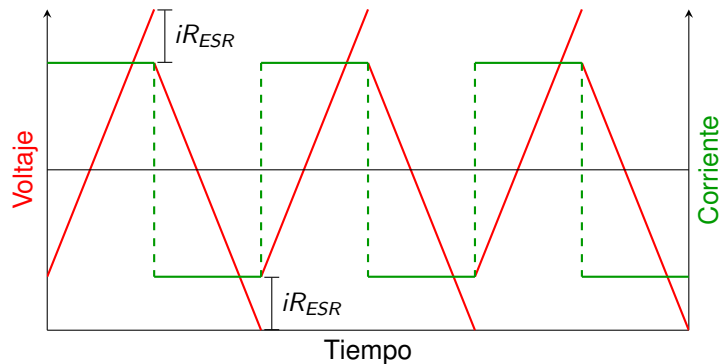
Figura 10: Carga y descarga de un condensador evidenciando el efecto de una ESR.
