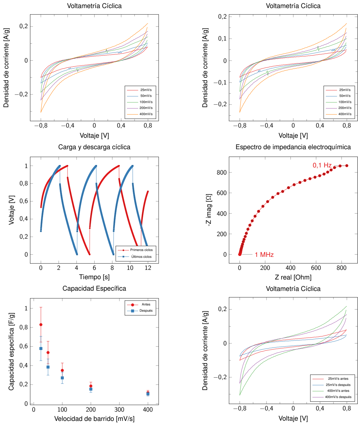
Figura A.9: Polvo en espuma de níquel. Masa = 0.9 mg..
