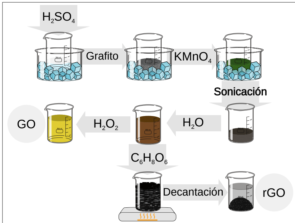
Figura 1.1: Método experimental simplificado para la síntesis de óxido de grafeno y óxido reducido de grafeno.
