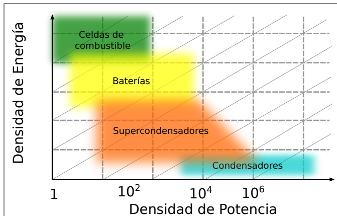
Figura 8: El diagrama de Ragone compara diferentes tecnologías de almacenamiento de energía de acuerdo a su densidad de potencia y densidad de energía.
