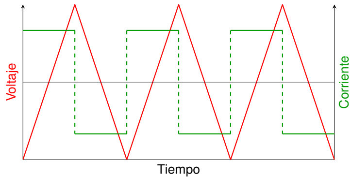
Figura 9: Carga y descarga de un condensador ideal a corriente constante.
