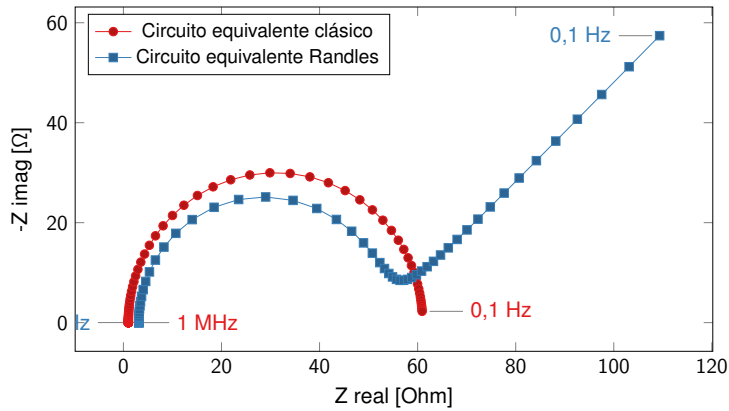
(c) Espectro electroquímico de impedancia simulados para los circuitos equivalentes (a) y (b). Obtenido en EIS Spectrum Analyser 6 .
