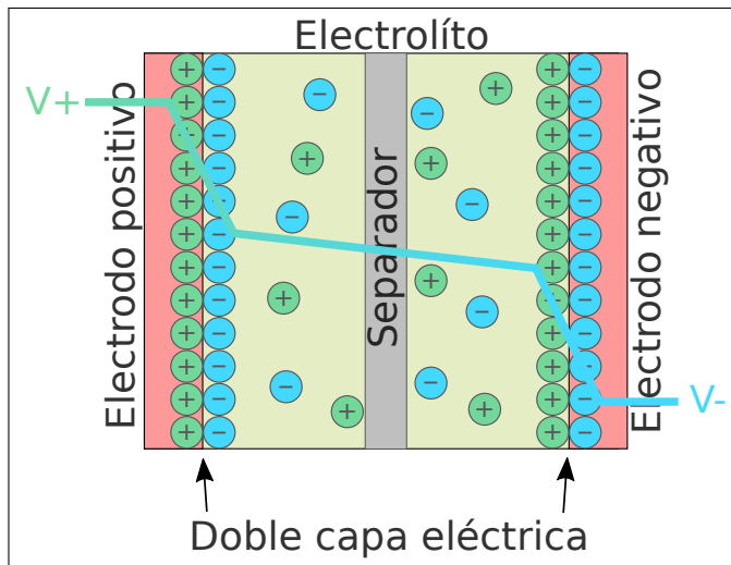
Figura 12: Esquema de un supercondensador mostrando una doble capa eléctrica de Helmholtz en cada electrodo y el perfil del potencial eléctrico en él.
