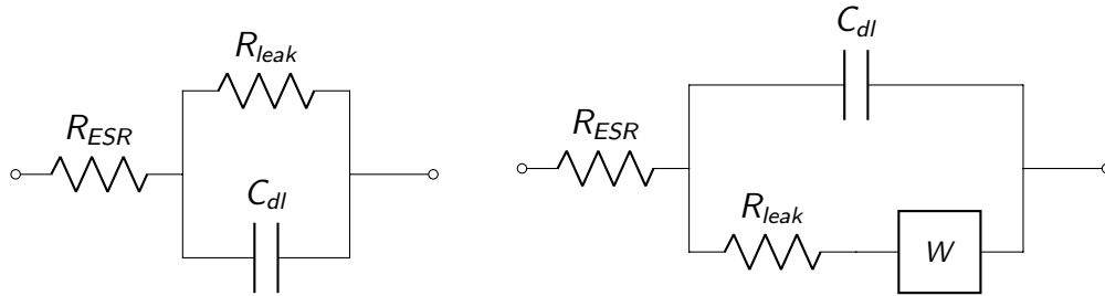
(a) Circuito equivalente clásico.
