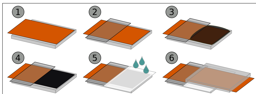
Figura 3.1: Secuencia para la construcción de un supercondensador básico.
