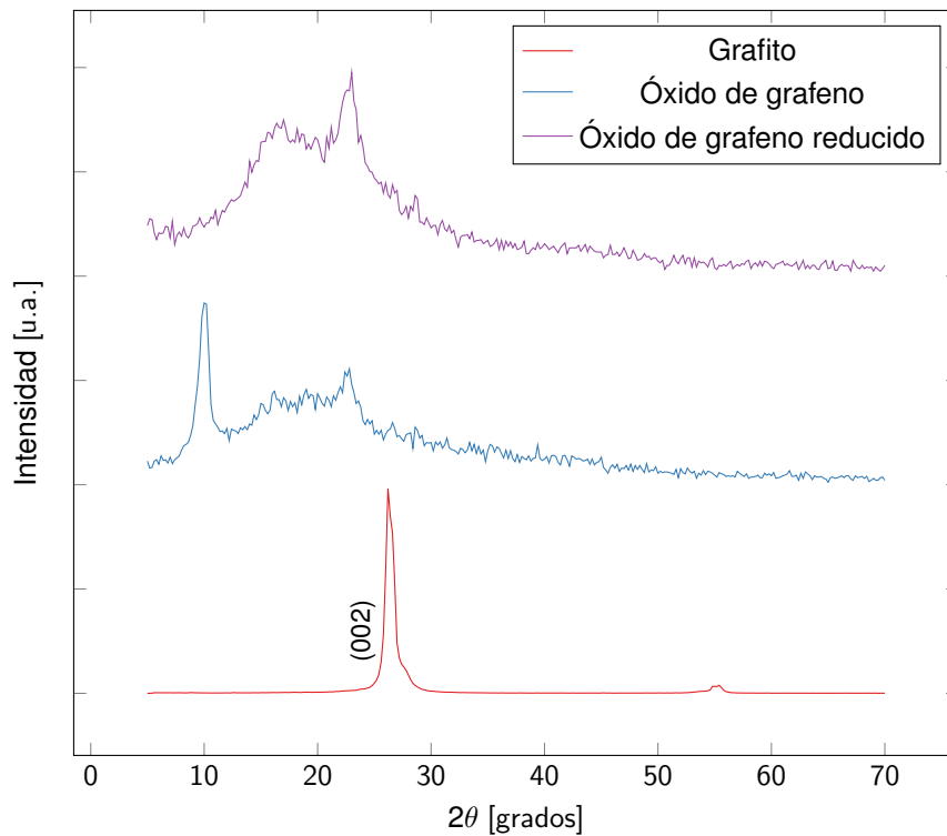
Figura 2.2: Espectro de difracción de rayos x.
