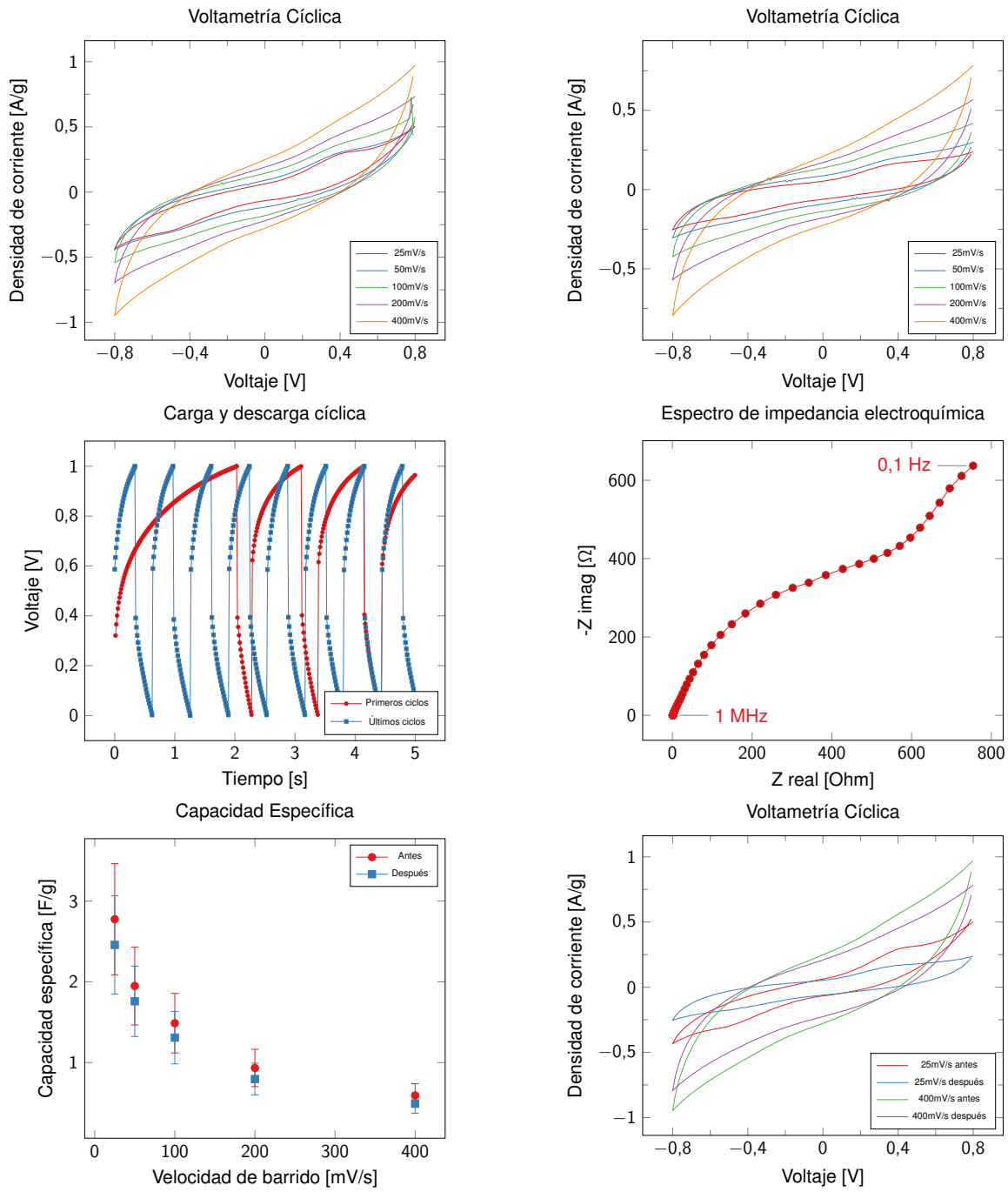
Figura A.10: Polvo + PMMA en espuma de níquel. Masa = 0.8 mg.
