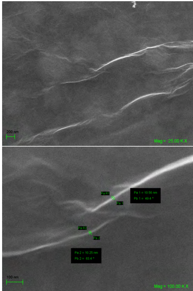
Figura 2.4: Imagen SEM de un electrodo de rGO en formato papel (PapelAc ).
