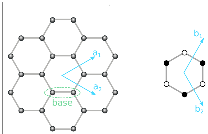
Figura 5: Izquierda: Red de grafeno en espacio real. Derecha: Red en espacio recíproco.
