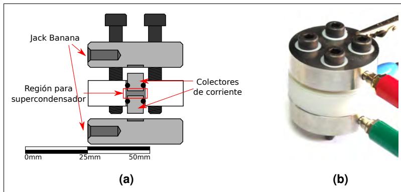
Figura 3.2: (a) Vista en corte longitudinal de la celda de pruebas mostrando los componentes más importantes. (b) Fotografía de la celda armada y conectada al potenciostato.
