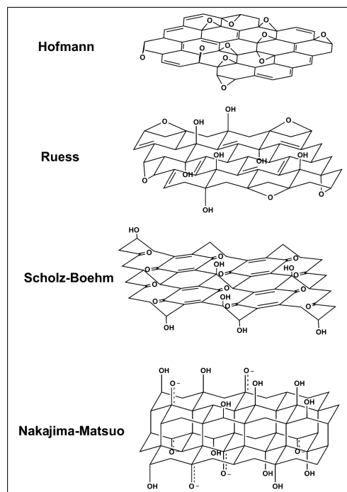
Figura 7: Estructuras propuestas para el óxido de grafeno (Dreyer et al., 2010).
