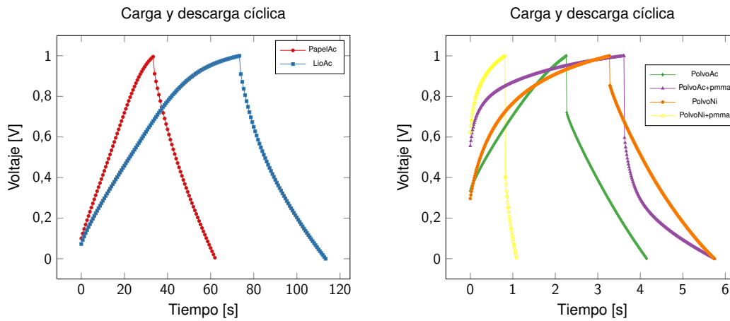
Figura 3.6: Resumen de carga y descarga cíclica a 1 A/g, exceptuando las muestras de polvo más pmma en disco de acero y polvo en espuma de níquel donde la densidad de corriente es de 0,1 A/g. Las muestras son separadas en dos gráficos para mejorar su visualización.
