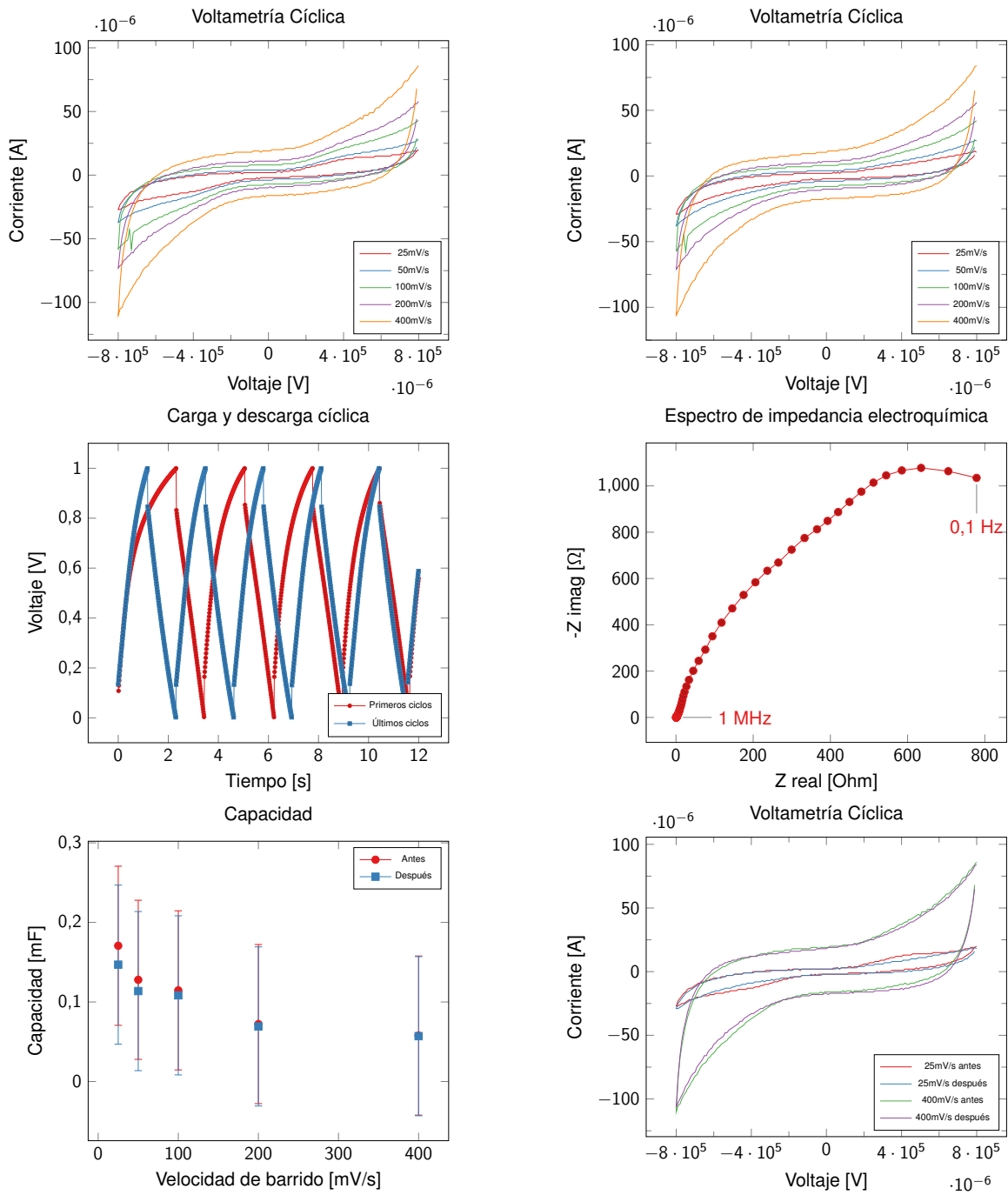
Figura A.8: Espuma de níquel sin material.
