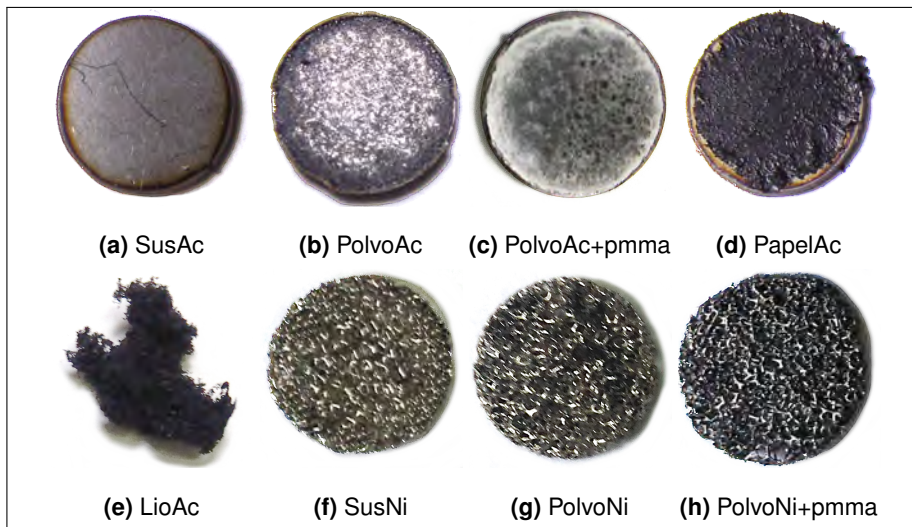
Figura 3.3: Electrodo utilizados en la celda de pruebas de supercondensador, nombrados por sus alias de la tabla 3.1. El electrodo LioAc de la figura (e), se introduce en la celda tal cual se muestra, procurando cubrir todo el sustrato de acero.
